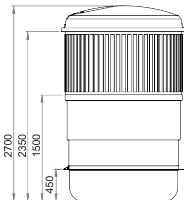
Boční pohled
