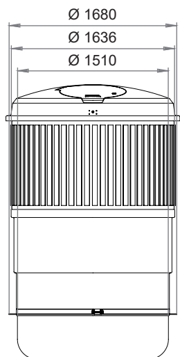
Čelní pohled
