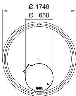
Horní pohled
